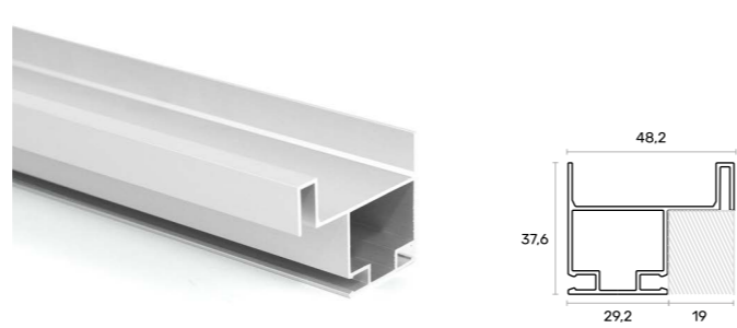
PERFIL GOLA LATERAL 800 SIDE VERTICAL 800 GOLA PROFILE
